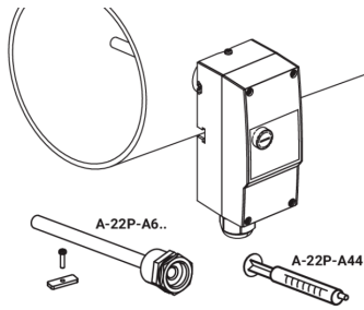
Tauchhülsenmontage
