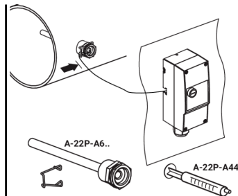
Wandmontage mit Sonde in der Tauchhülse
