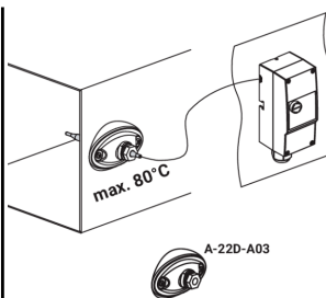
Wandmontage mit Sonde im Flansch
