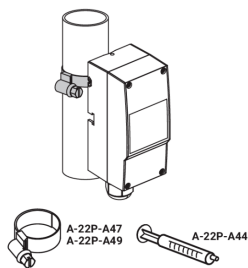
Rohr-Anlegemontage
