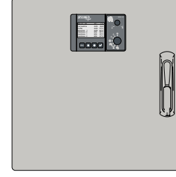
1-fach QDR - mit / with Montageplatte / Mounting plate 450x450x200mm Bestellnummer / Order Number: 400.15894
